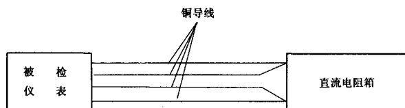
(a) 配三线制热电阻
