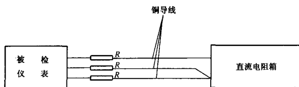
(a) 配三线制热电阻
